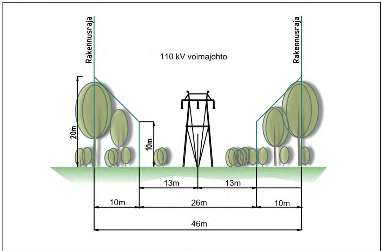
Kuva 13. 110 kV voimajohtoon tyypipoikkileikkaus.
